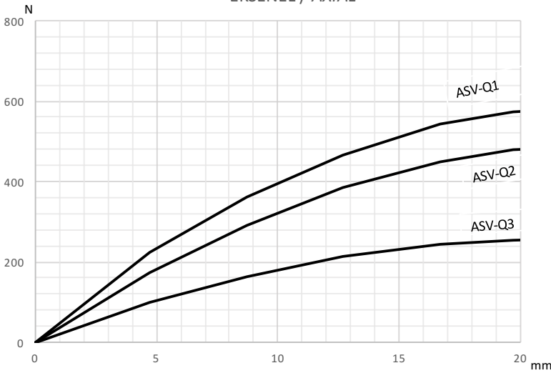
EKSENEL / AXIAL
